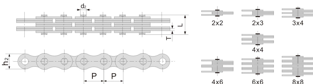
Plate structure 链板组合
